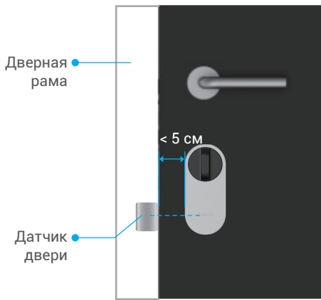
Вид спереди
