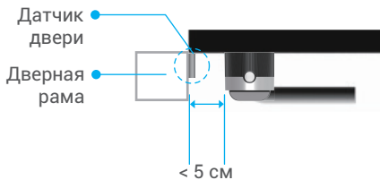
Вид сверху
