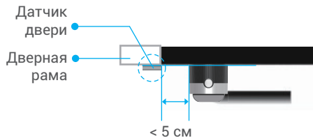
Вид сверху
